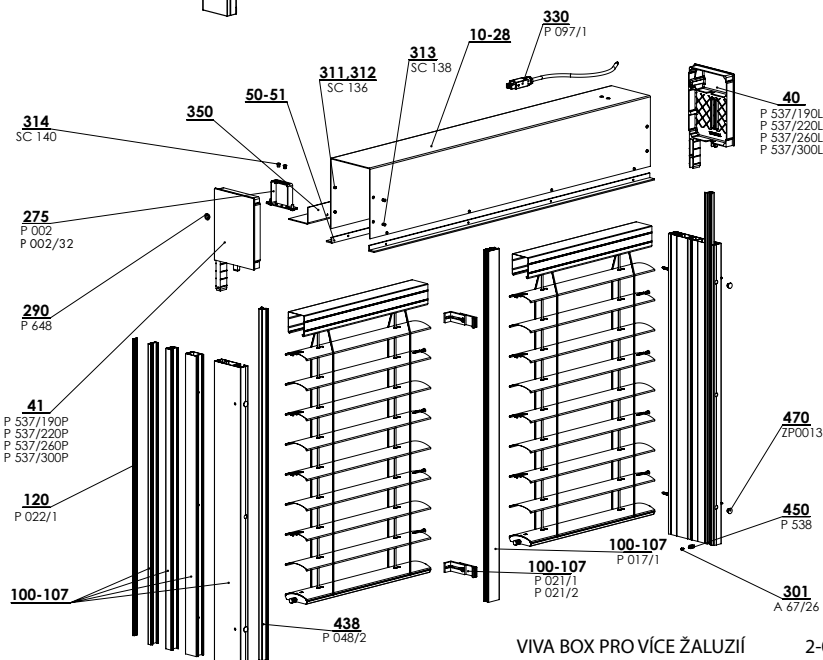
KASTLÍK PRO SAMONOSNOU VŽ (vodící lišta RS75) 2-01016-XXXX-D
